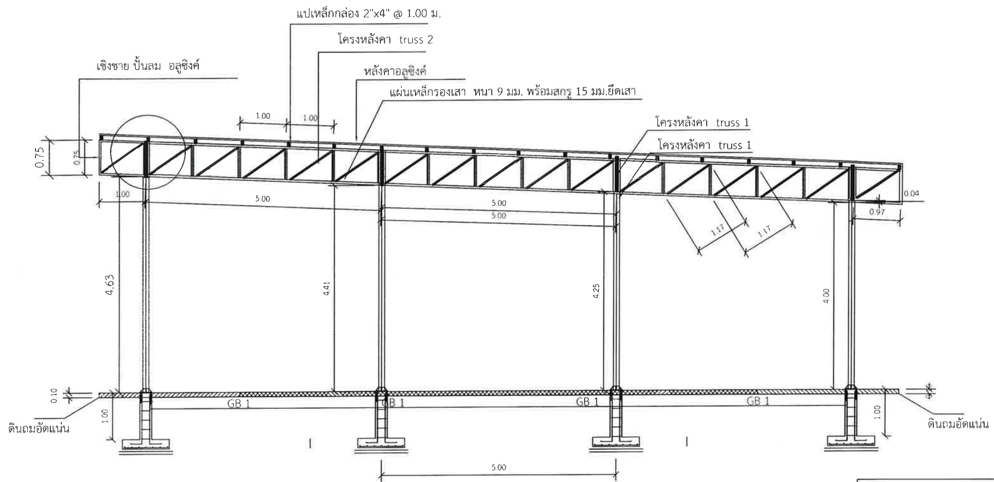
รูปตัดตามขวาง
