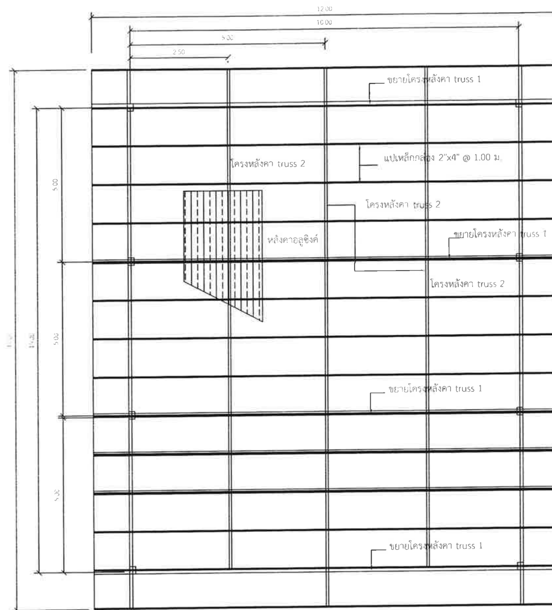
แบบอนโครงหลังคา
