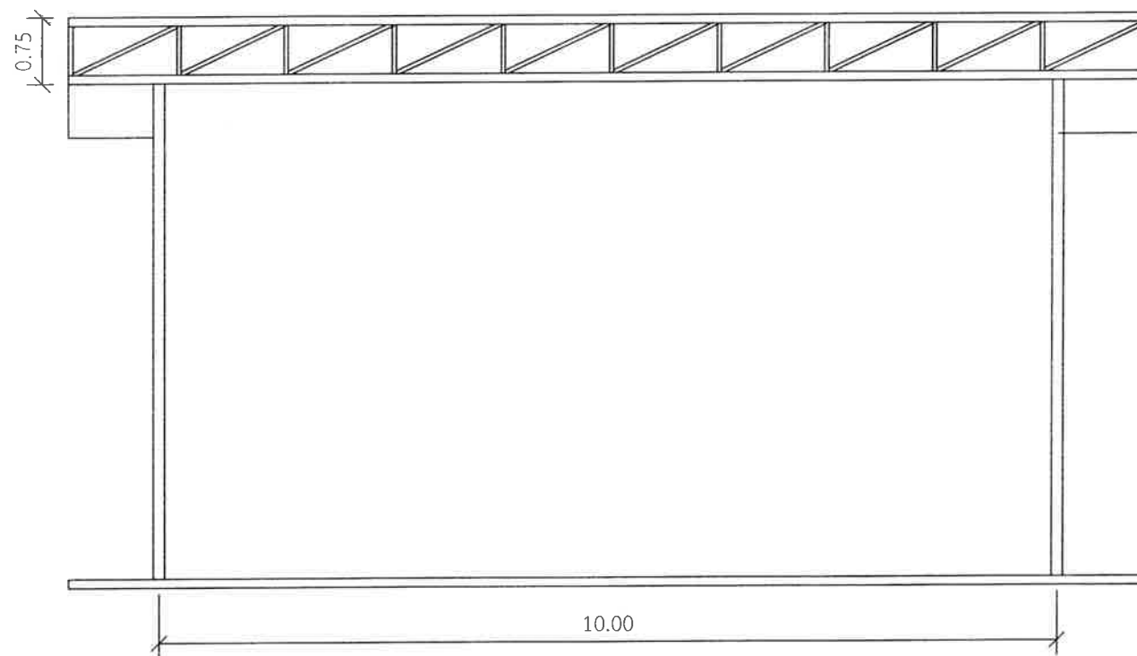
รูปตัดด้านหน้า
