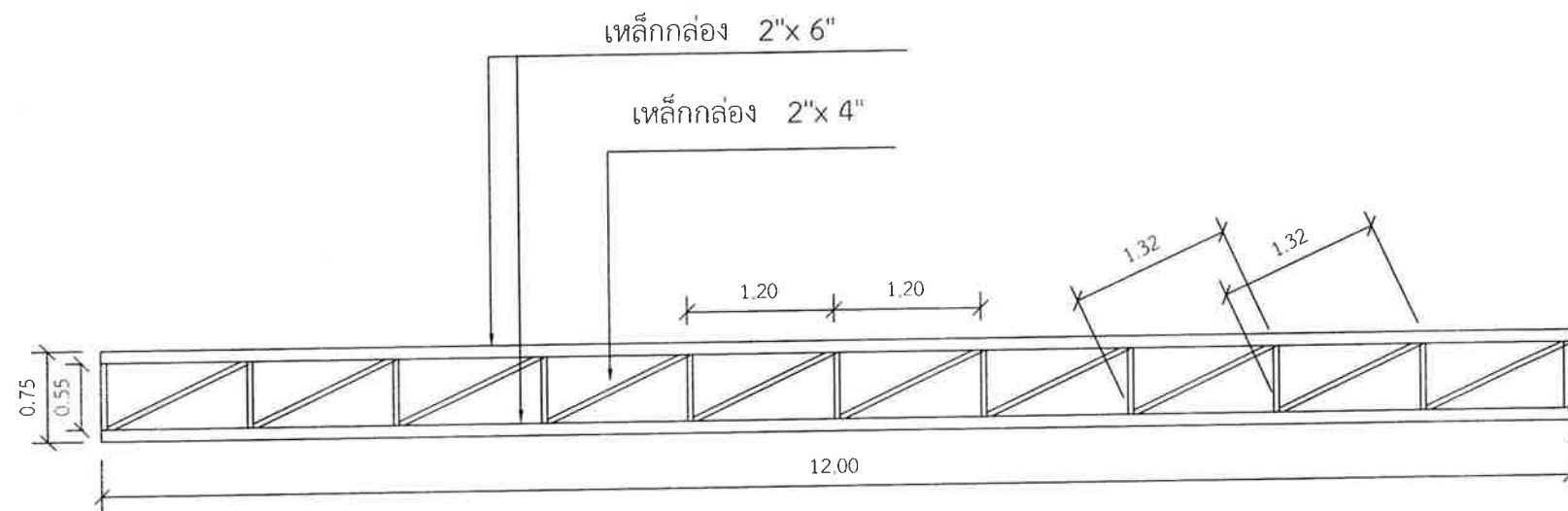
ขยายโครงหลังคา truss 1
